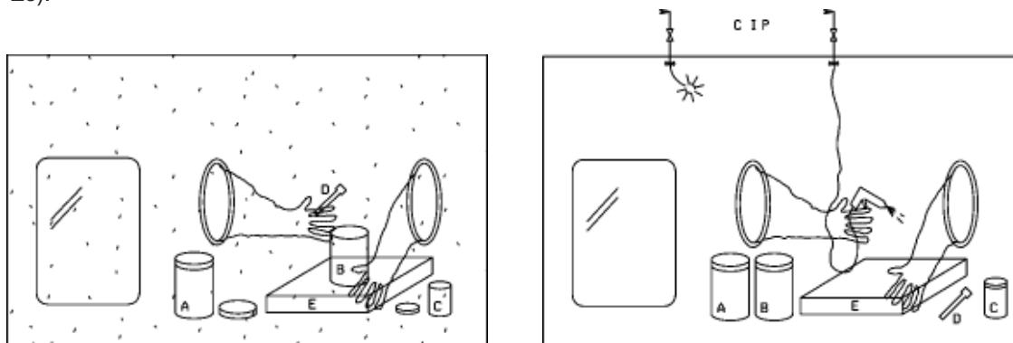
Figure 28-29. - Isolatore a camera singola che richiede la bonifica completa prima della riapertura della porta
